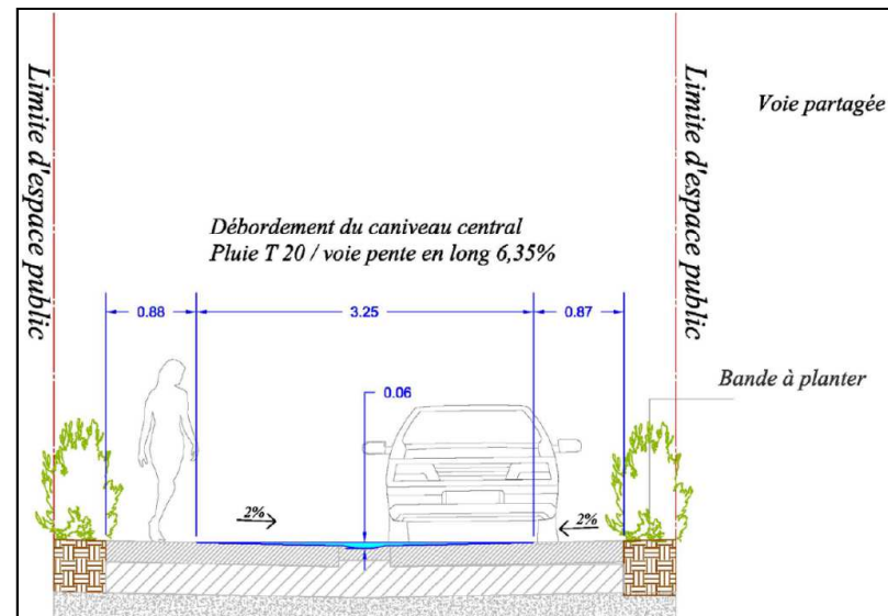
Coupe de la collecte sur voirie sans noue
